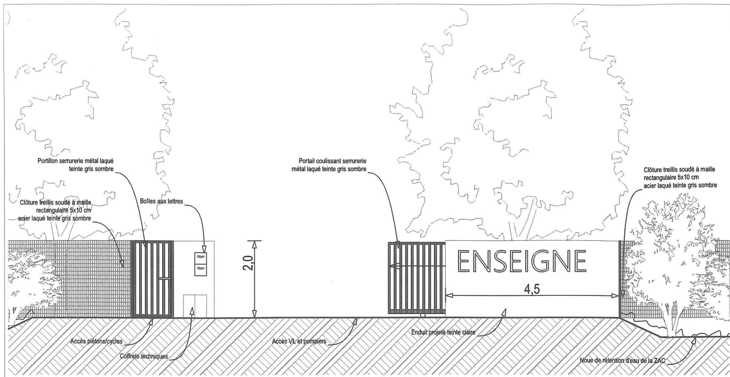
ENTREE PRINCIPALE DES LOTS / MURET TECHNIQUE - épaisseur 20cm / ECH 1-100
